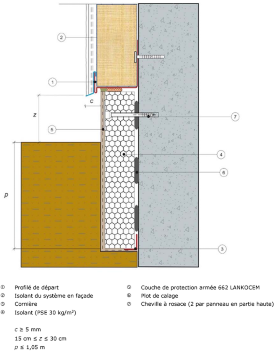
Figure 4b : Départ sur isolant en partie semi-enterrée – pose calée-chevillée Figure 4 : Traitements en partie semi-enterrée
