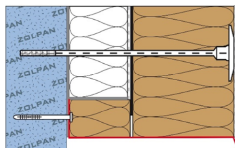
Figure 2c : Ancien profilé disqué Nouveau profilé standard
